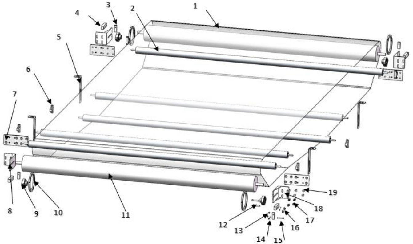
毛毡滚动部件
