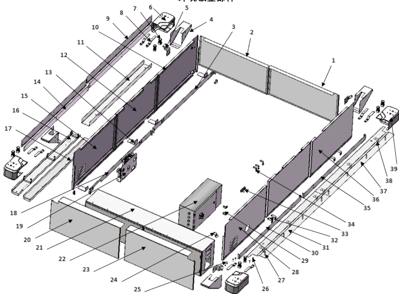
外观钣金部件
