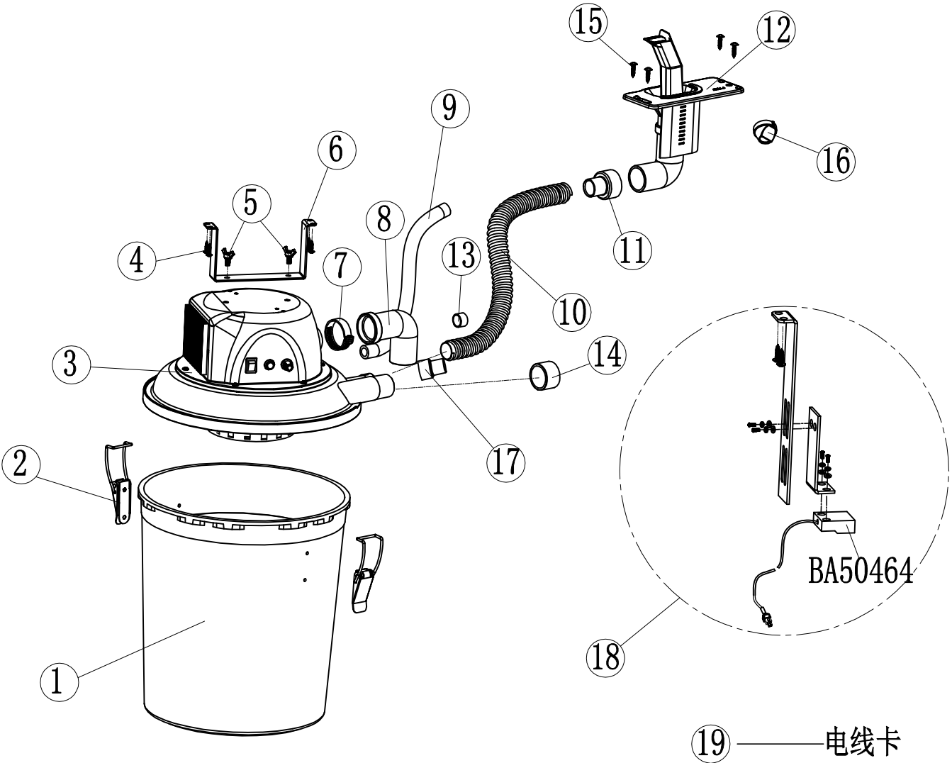
BA1600D无刷一体式集尘装置装配图
