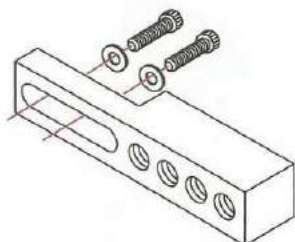
Bracket for Pfaff machines 百福機型用轉接配件
