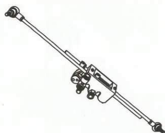
Heel action switch 腳跟後踏拉桿
