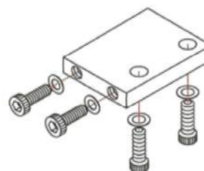
Bracket for Durkopp Adler 195, 243, 244, 291, 294, 296, 491 杜克普 195, 243, 244, 291, 294, 296, 491 用轉接配件
