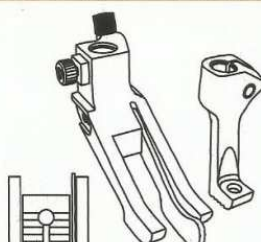
Right guide feet 右傍壓腳
