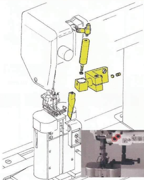
Pneumatic guiding set for Juki PLC-1760 重機1760 氣動傍位
