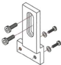
Bracket for Durkopp Adler 204-370, 205-370 杜克普 204-370, 205-370 用轉接配件
