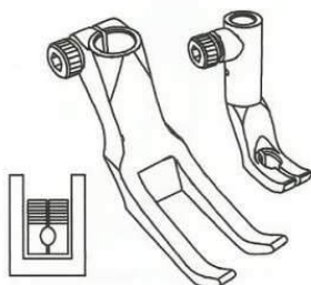
Regular foot 標準壓腳
