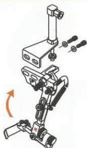
Pneumatic lifted edge guide 泛用型氣動升降傍位
