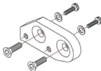
Bracket for Durkopp Adler 267, 268, 269 杜克普 267, 268, 269 用轉接配件
