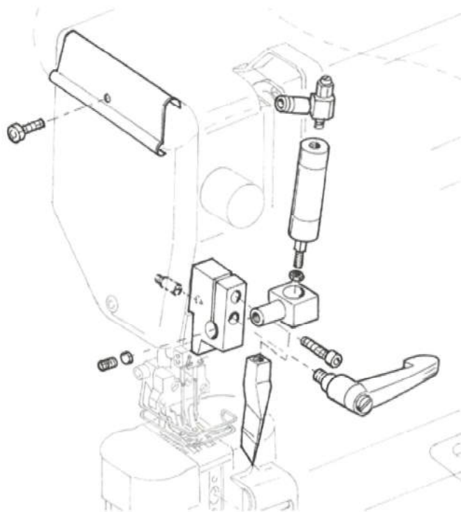
Pneumatic guiding set for 768 768 氣動傍位
