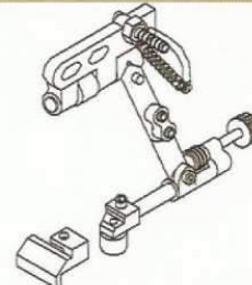
Zipper guide & 14mm diameter roller guide 拉鏈傍位及14mm直徑滾輪傍位
