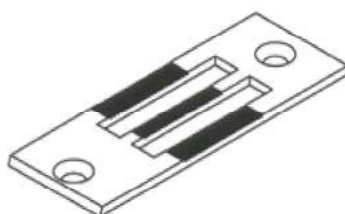
Needle plate 針板
