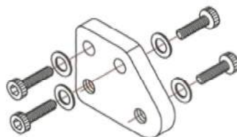
Bracket for Durkopp Adler 669, 867, 868 杜克普 669, 867, 868 用轉接配件
