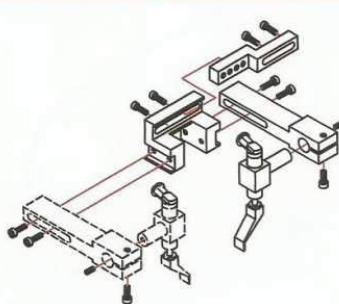
Pneumatic guide 泛用型氣動傍位
