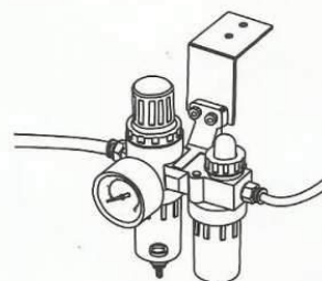
F.R.L. Unit - Filter, Regulator, Lubricator F.R.L. 聯組 - 減壓閥、壓力表、油霧器
