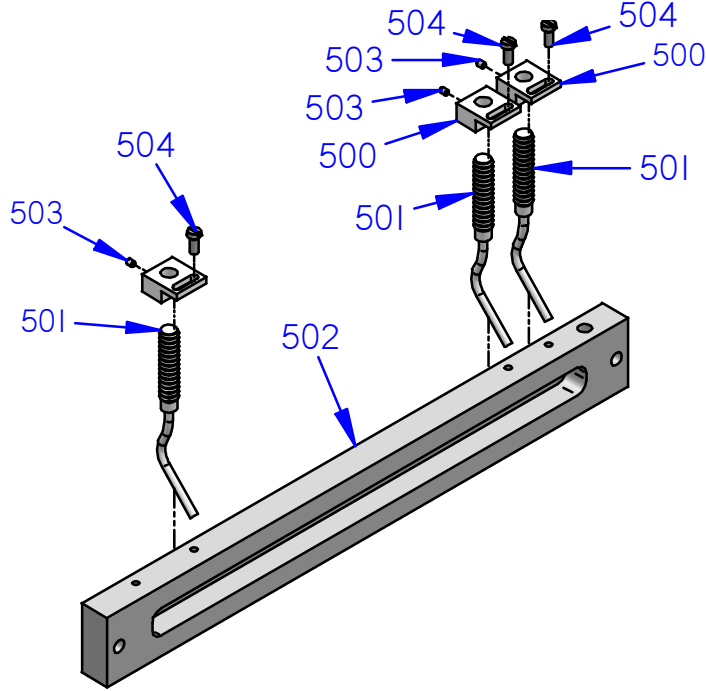
2650K514 GRUPPO BASE CARICA PASSANTE
