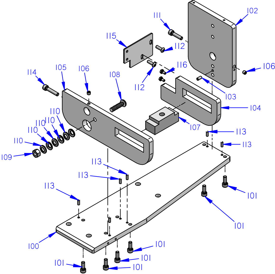
2650K514 GRUPPO BASE CARICA PASSANTE
