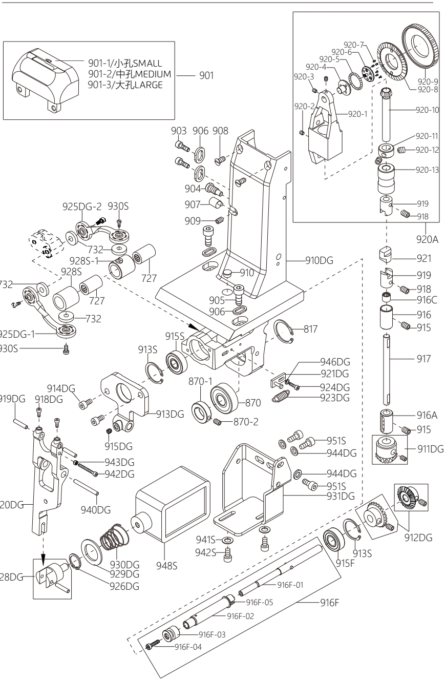
9 单针中座及下倒缝机构（短线头）
