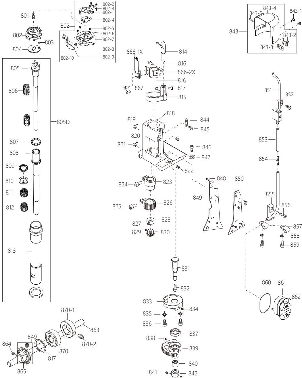
8 右边座机构（短线头） Right side bracket mechanism
