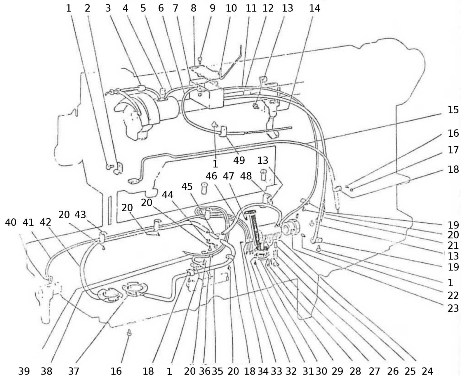
MECCANISMO LUBRIFICAZIONE OLIO
