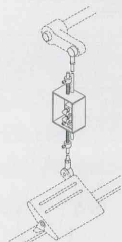
AF 腳踏開關 Pedal switch
