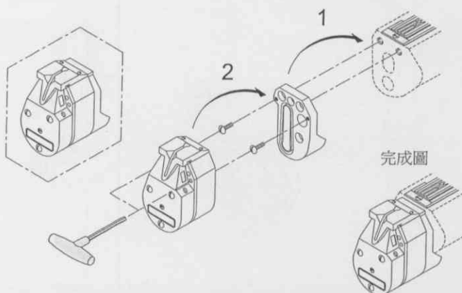
安裝EFV Install EFV
