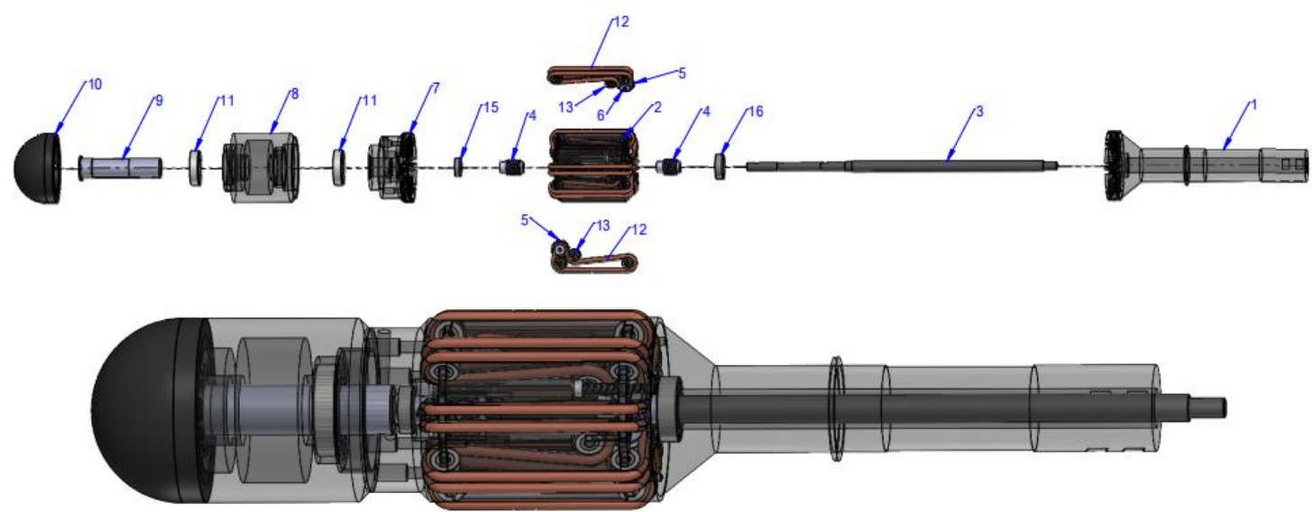
QK300H-06-000-1B 纠偏轮组件
