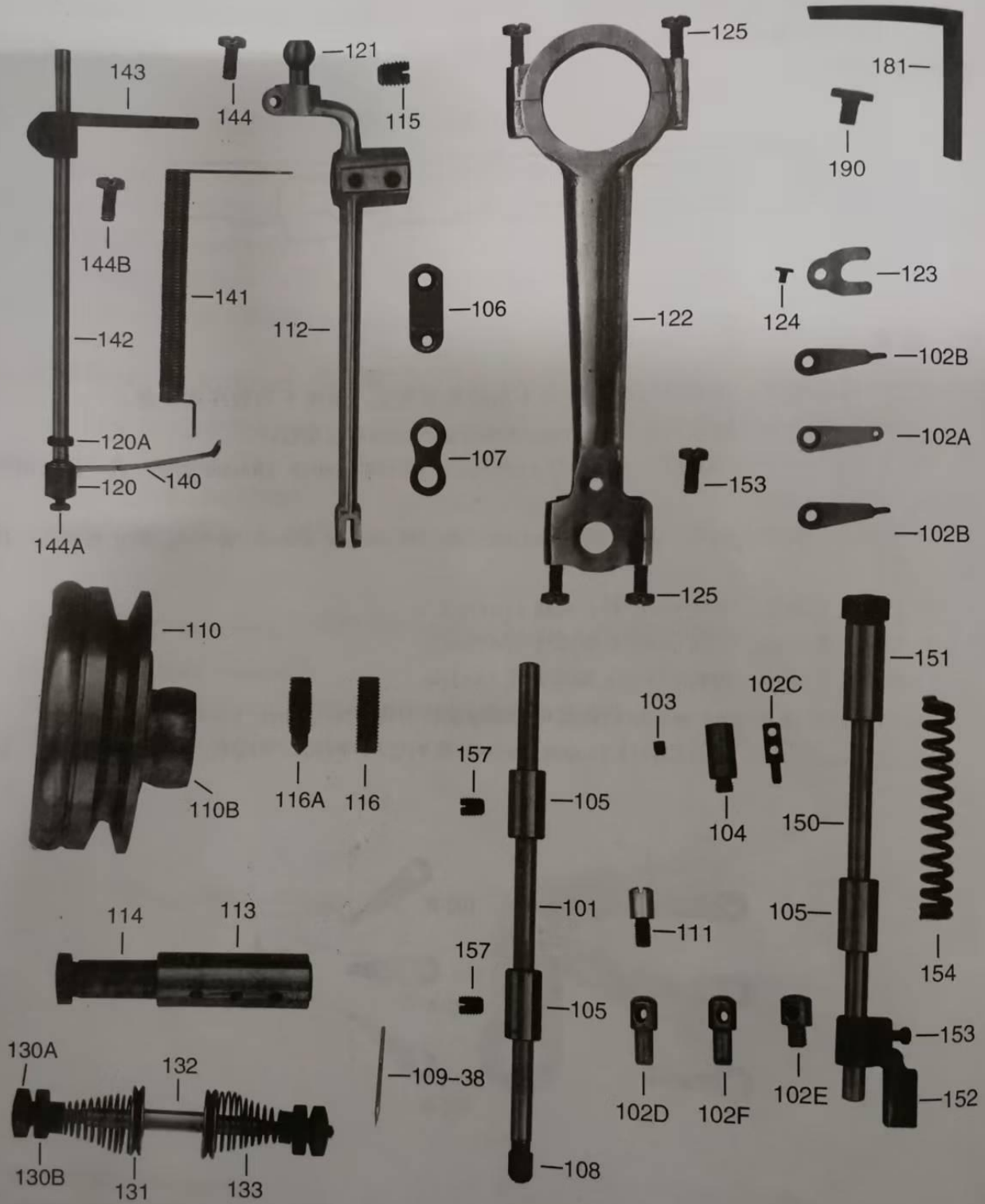
零件图(1)
