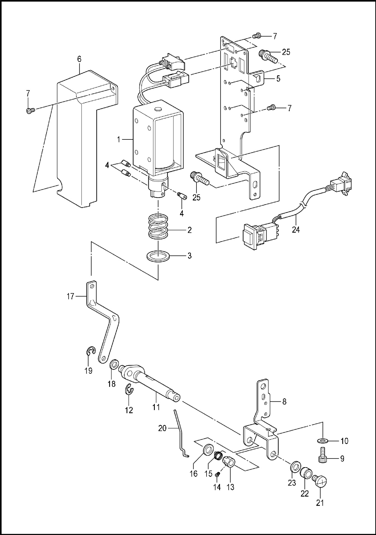
K . 扫线装置 / Thread wiper mechanism
