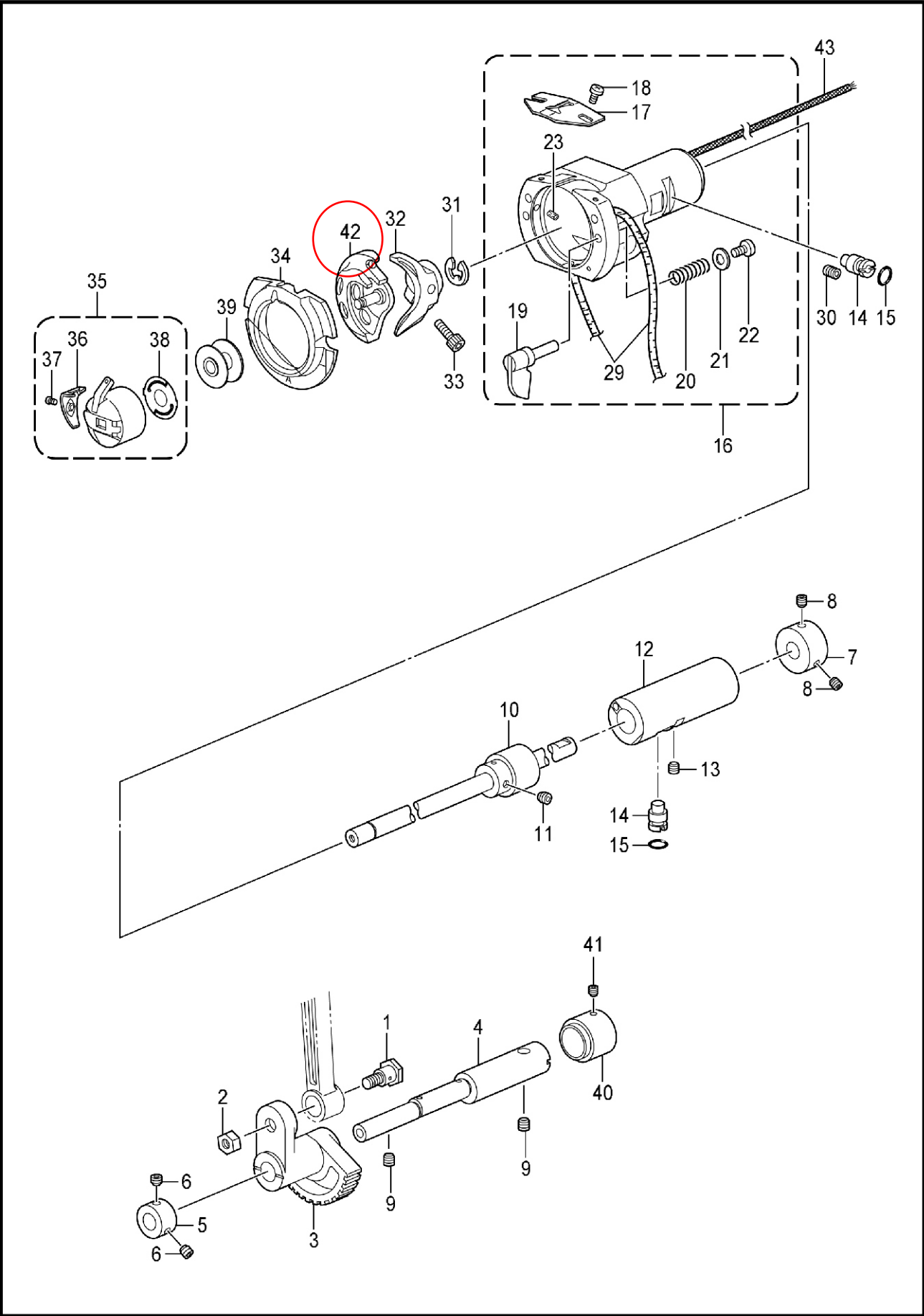
E. 下轴装置 / Lower shaft mechanism
