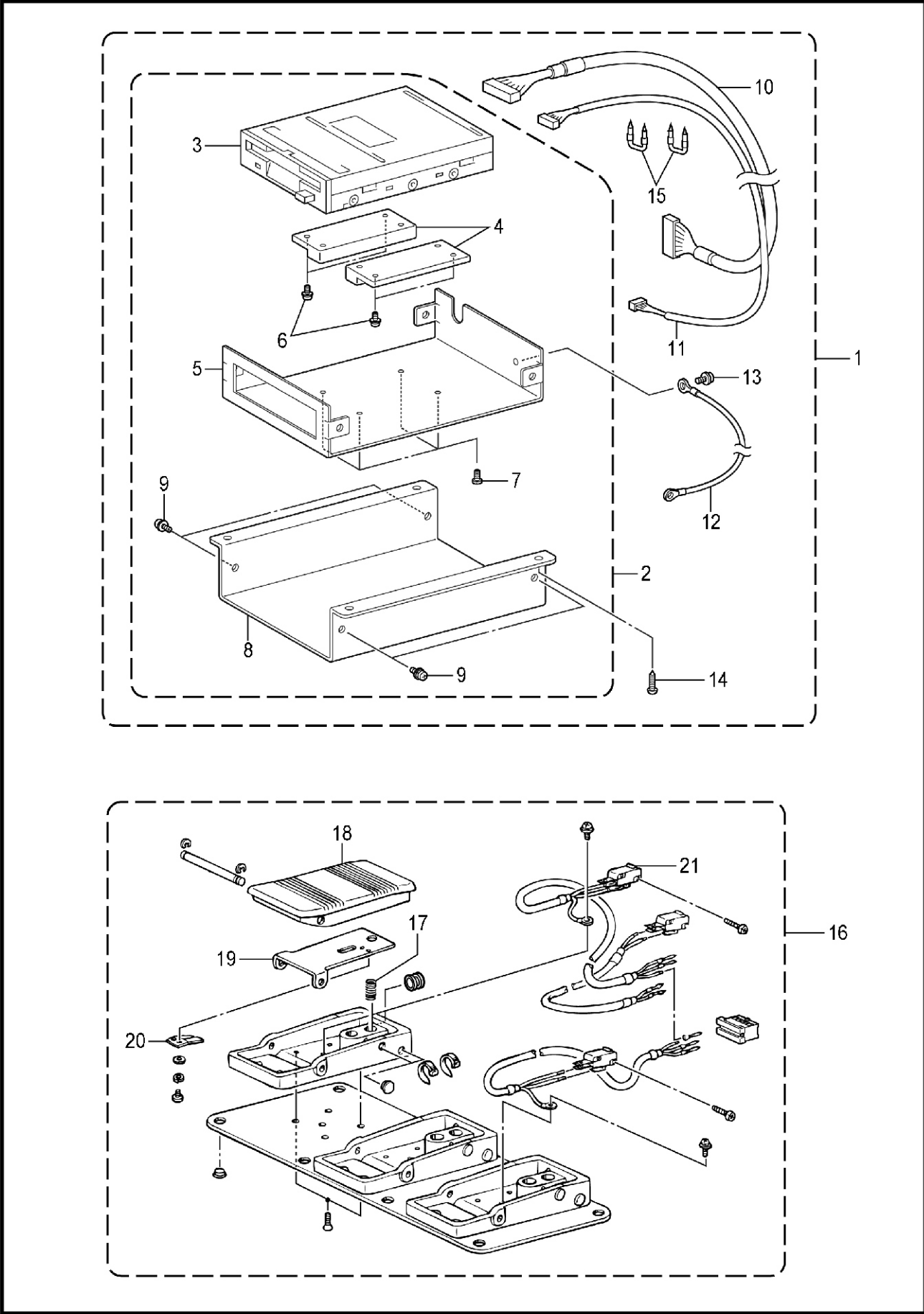
V2 . 附属装置(选购件) / Attachment set (Option parts)
