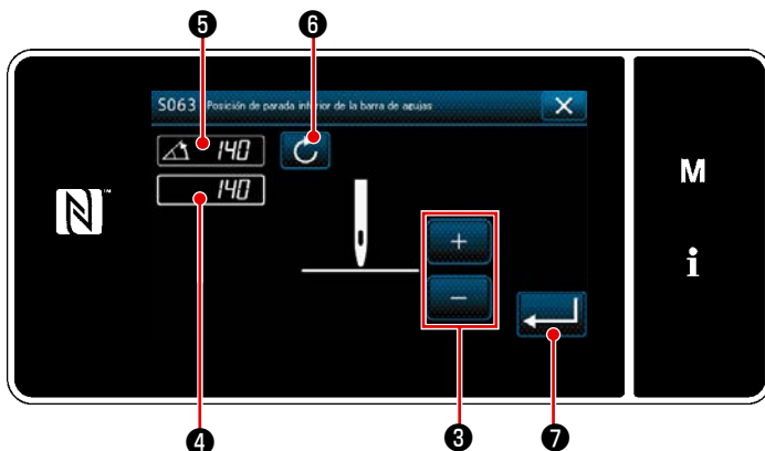
<Pantalla de ajuste de posición de parada inferior de la barra de agujas>
