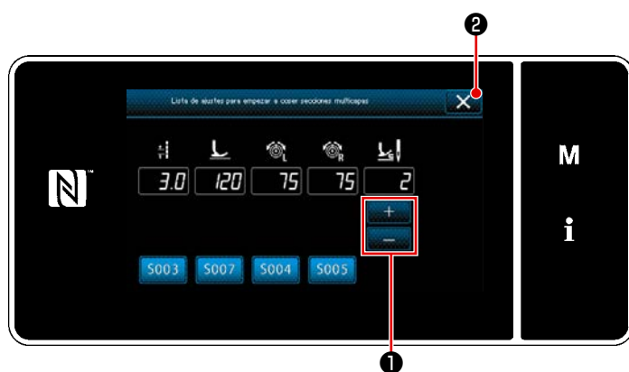
<Pantalla de la lista de ajustes de avance de sección multicapa>
