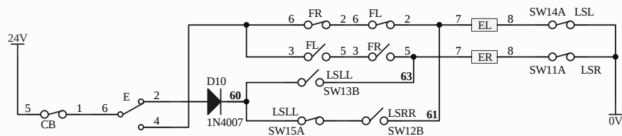
对边电机限位控制线路 EDGE SWITCH CONTROL
