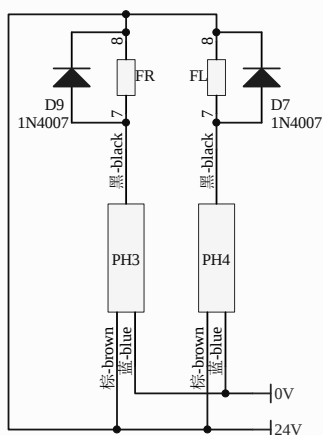
对边光电传感器控制线路 EDGE SENSOR CONTROL
