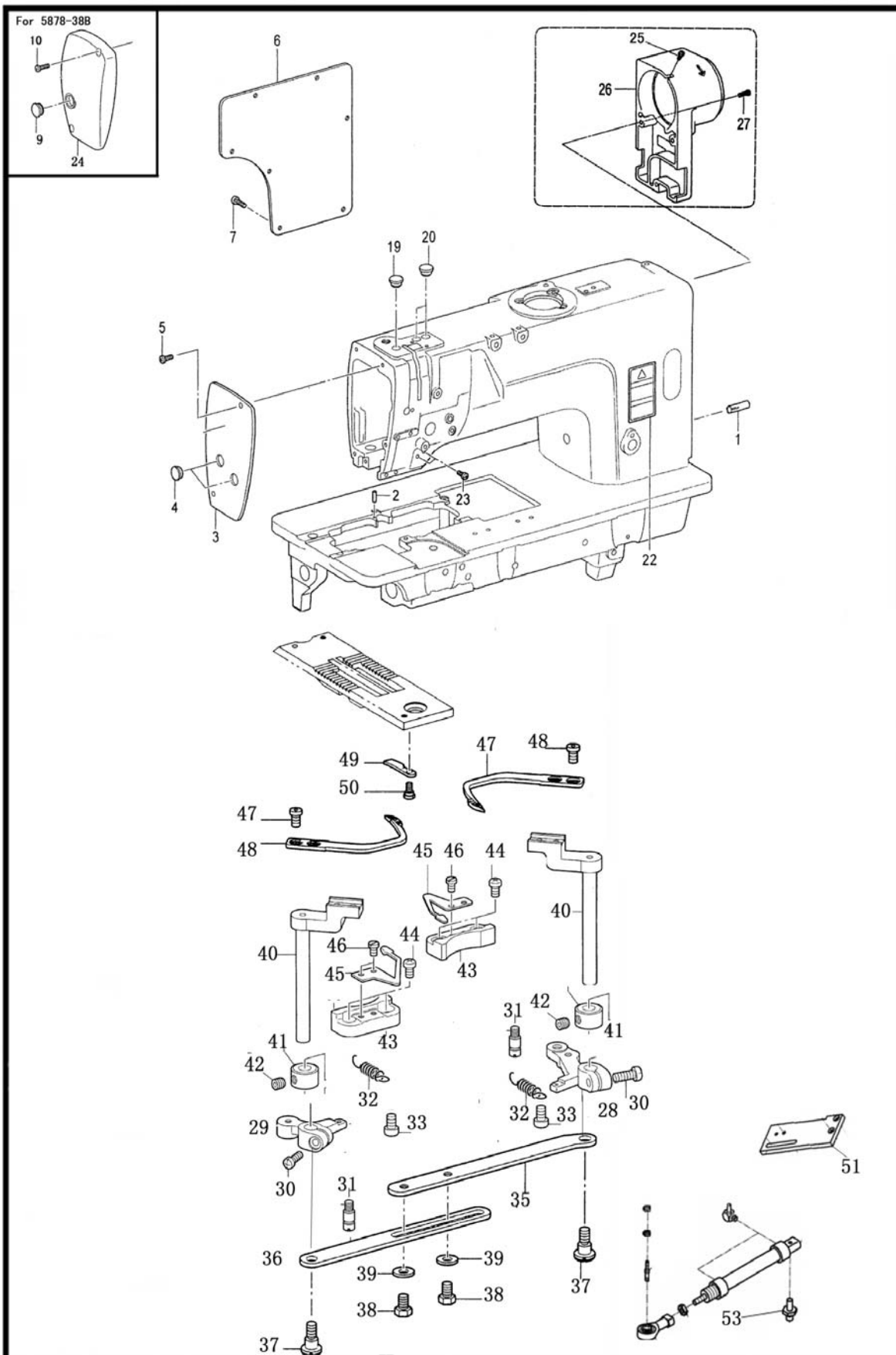
二十六 机头 & 剪线机构 平缝自动开袋机 Group 26 HEAD&TENSION TRIMMER FLAP POCKET MACHINE
