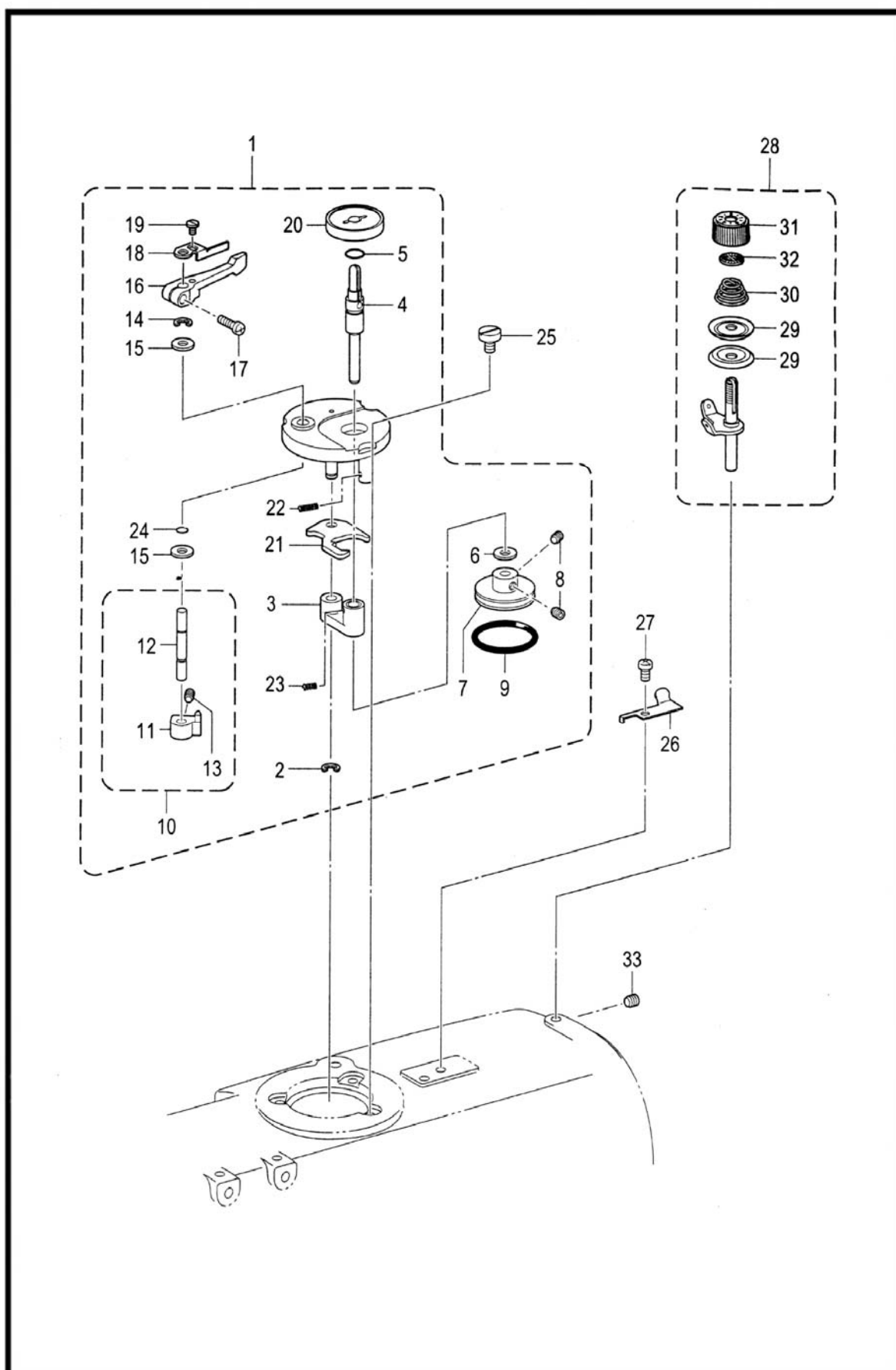
三十一 绕线机构 平缝自动开袋机 Group31 BOBBIN WINDER MECHANISM FLAP POCKET MACHINE
