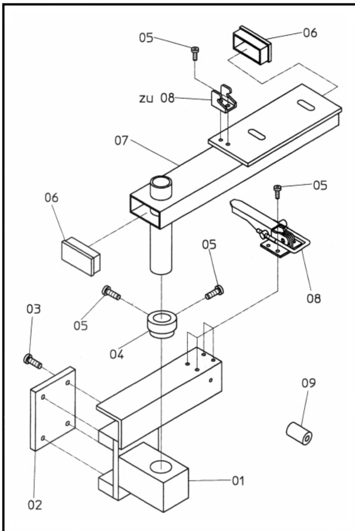
二十五 堆叠器连接臂 平缝自动开袋机 Group25 STACKER CONNECTOR ARM FLAP POCKET MACHINE
