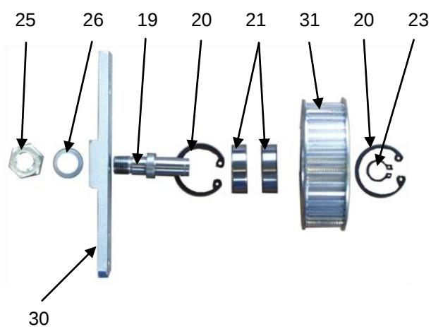
Tensioner pulley Item: 115410
