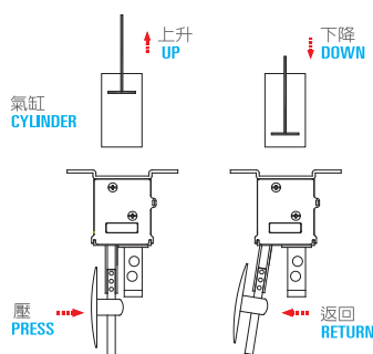
動作圖示 ACTION DIAGRAM
