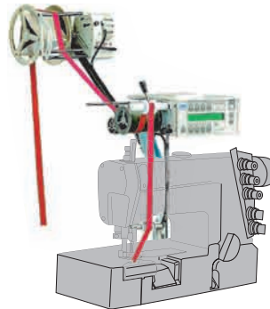
例二：飾縫車 EXAMPLE 2: COVERSTITCH
