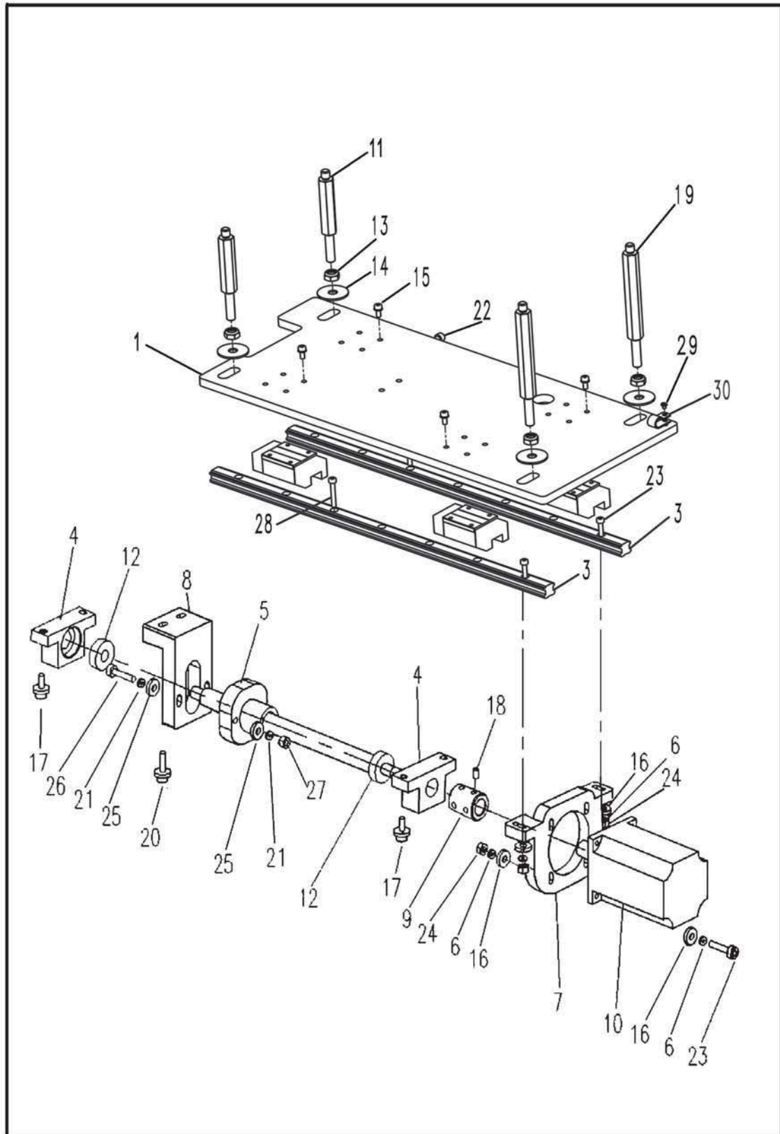
二 Group2 传动机构 TRANSMISSION MECHANISM 全自动门襟缝纫机 AUTOMATIC PLACKET SETTING MACHINE
